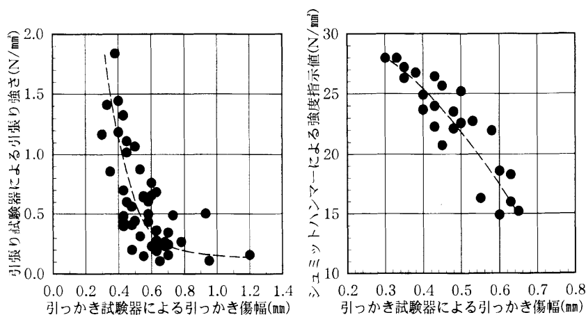
付図4 引張り試験器、シュミットハンマーと引っかき試験器による測定結果の関係 4)
