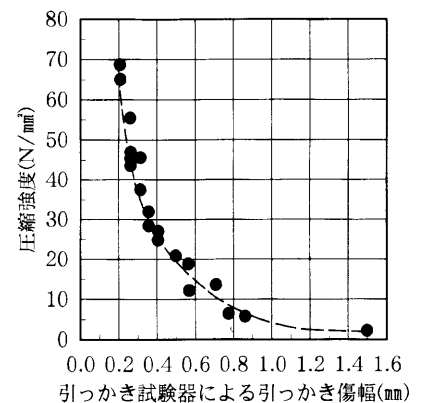
付図3 圧縮強度と引っかき傷幅の関係 3)
