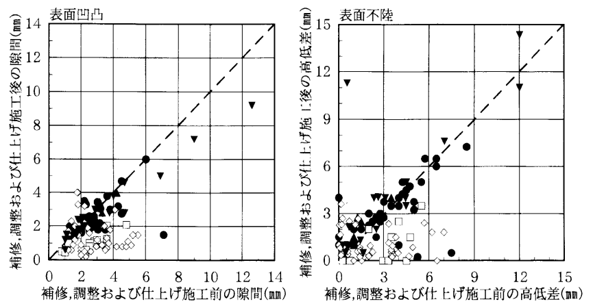
付図2 補修、調整および仕上げ施工前と施工後の隙間、高低差の関係
