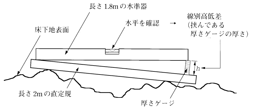
図3 不陸の測定方法
