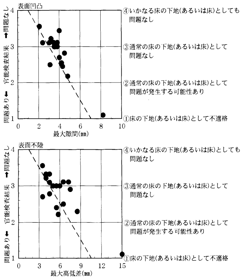
付図1 表面凹凸、不陸に関する官能検査結果と最大隙間、最大高低差の関係
