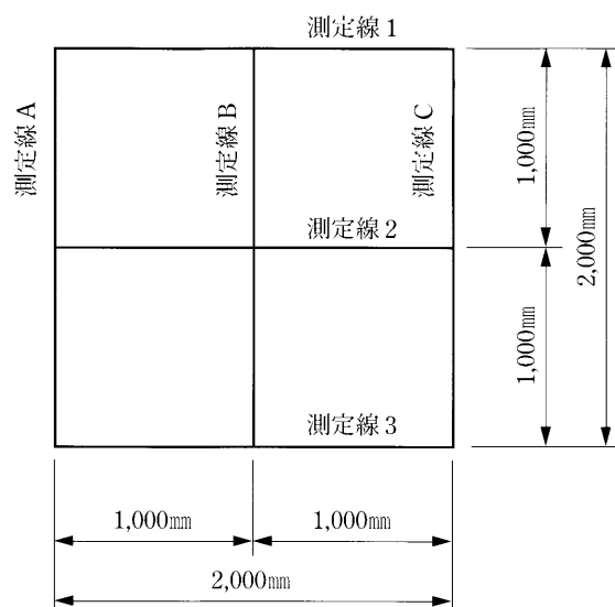
図1 測定線の設定方法
